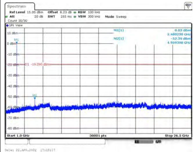
GFSK 2M
