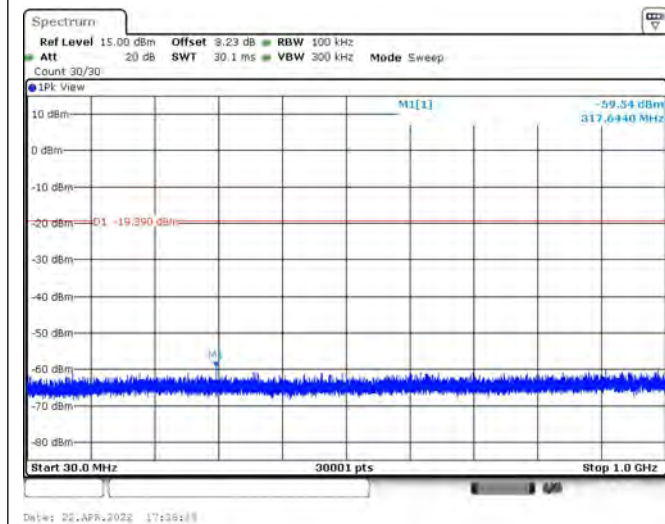
GFSK 2M
