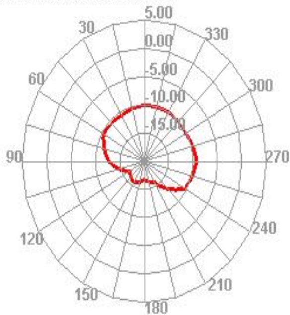
2405.000MHz H
