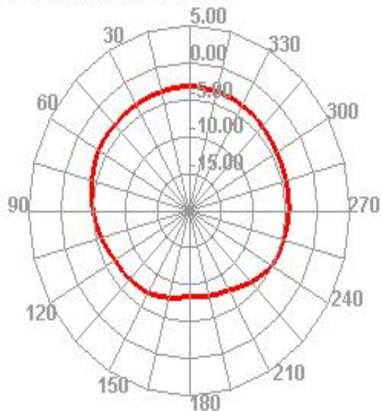
2480.000MHz H
