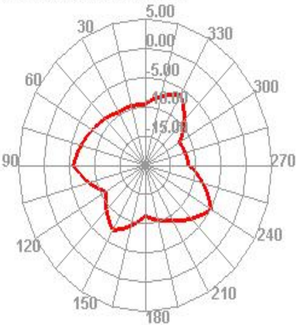
2450.000MHz E1
