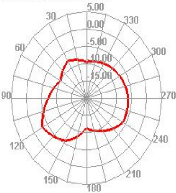
2450.000MHz E2
