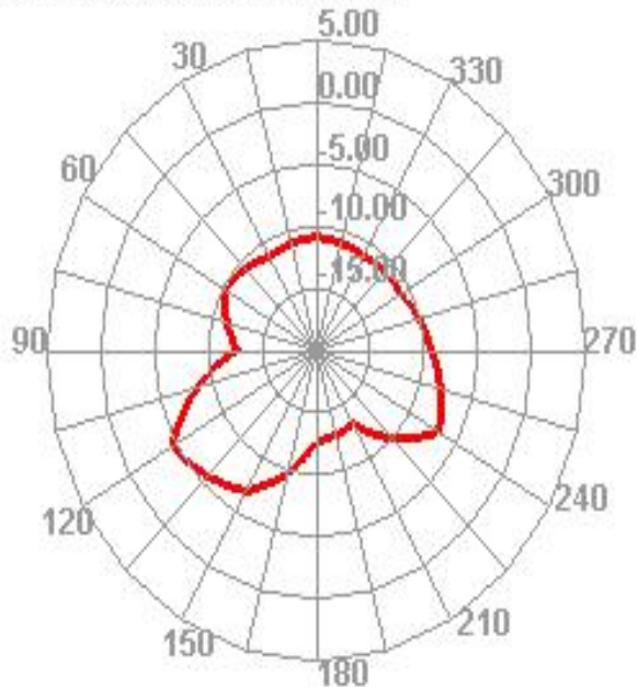
2405.000MHz E2
