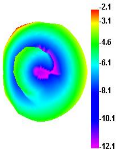
2480.000MHz
