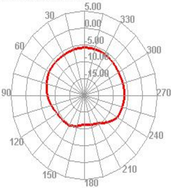
2450.000MHz H
