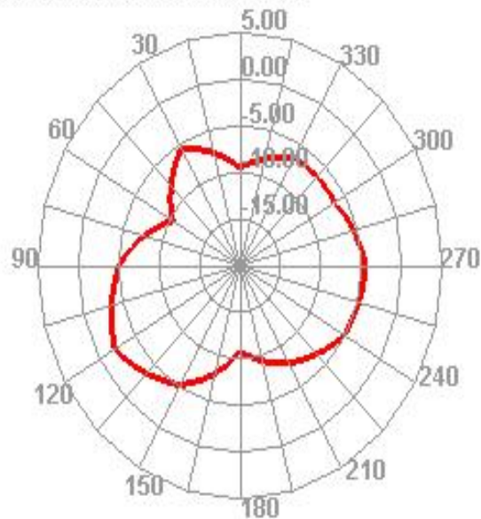
2480.000MHz E2
