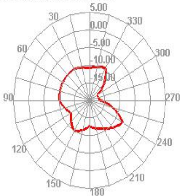
2405.000MHz E1
