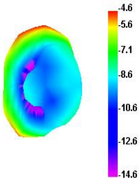
2405.000MHz
