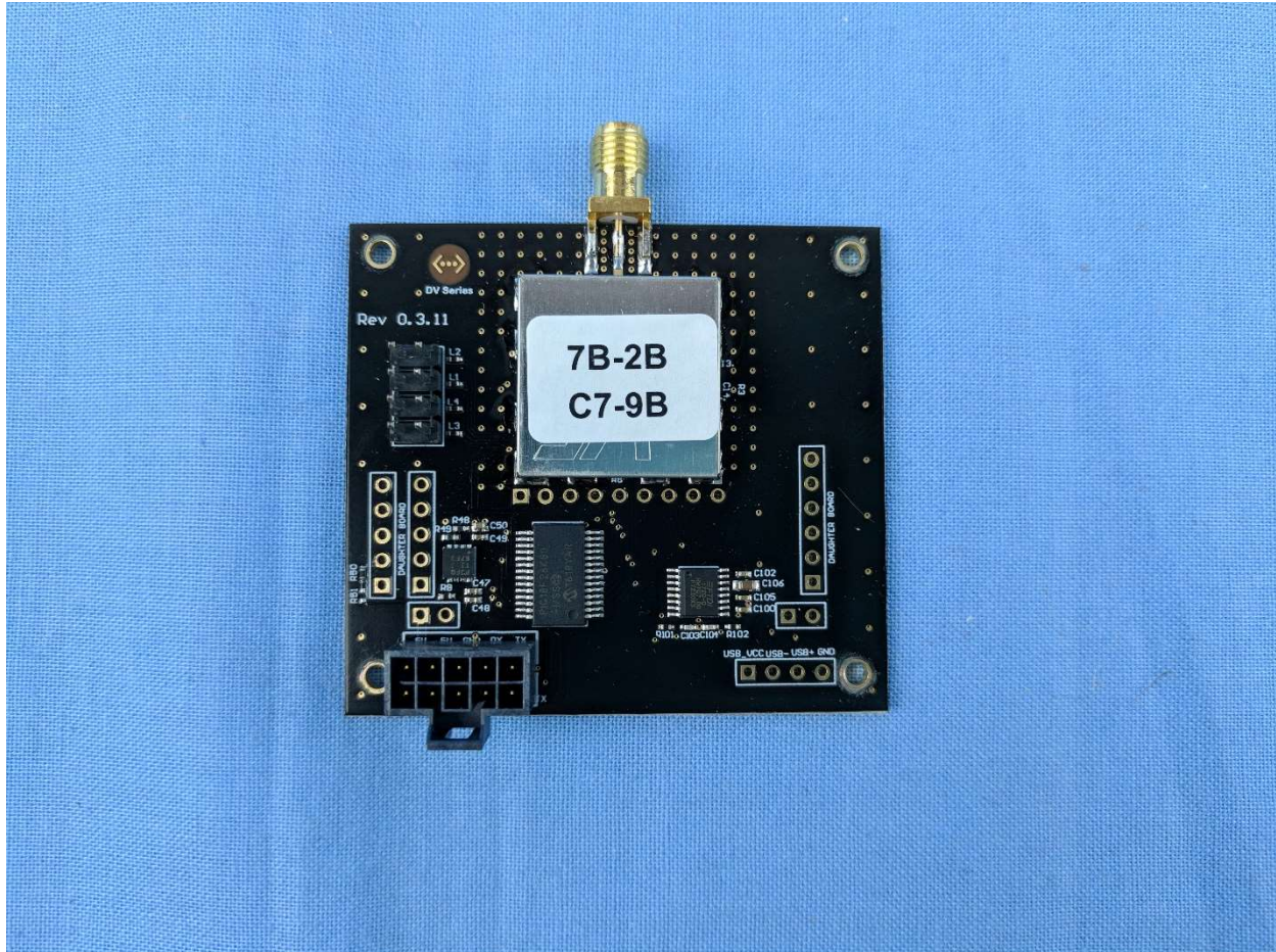
Module Top
