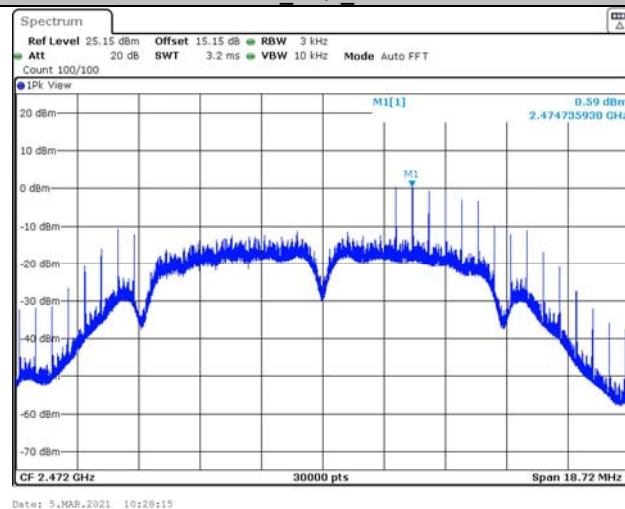
11B_Ant1_2472
