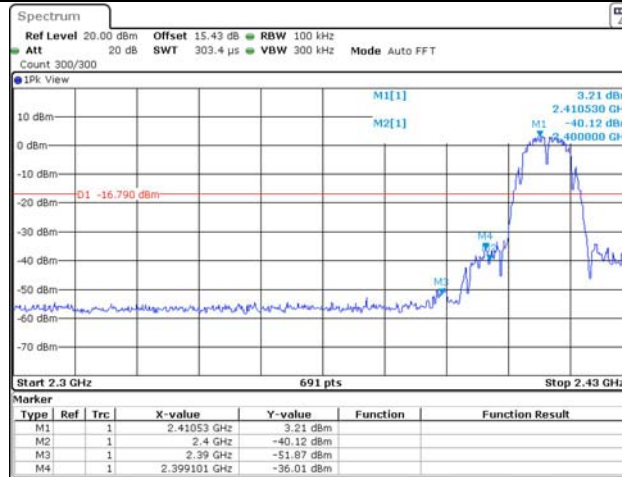
11B_Ant1_Low_2412
