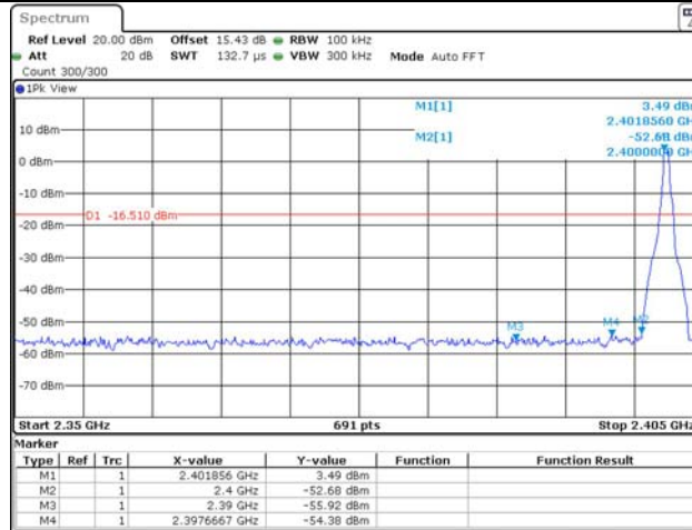
DH1_Ant1_Low_2402
