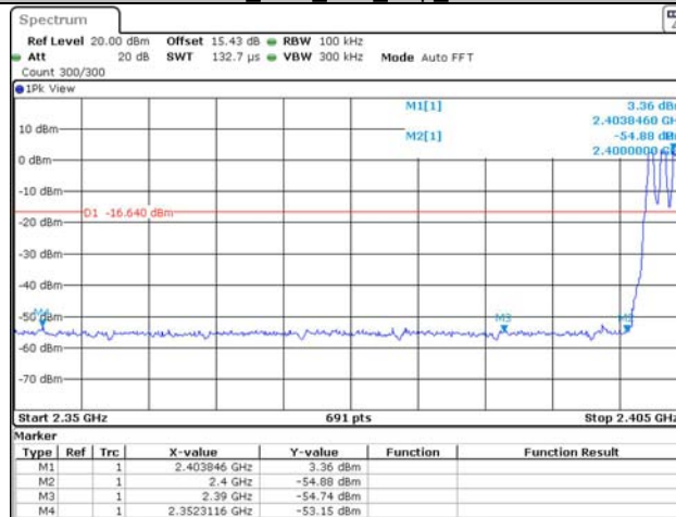
DH1_Ant1_Low_Hop_2402
