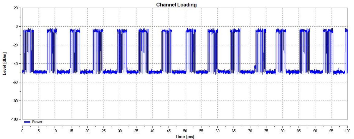
IEEE 802.11n HT20
