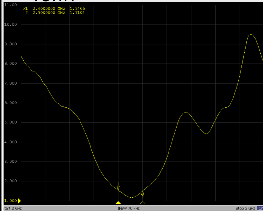
VSWR
