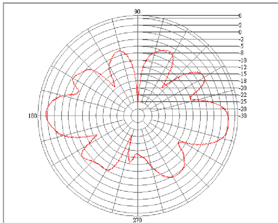
E-Plane 900mhz
