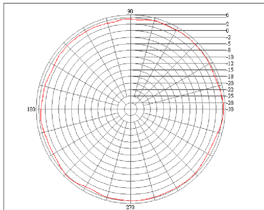
H-Plane 900mhz
