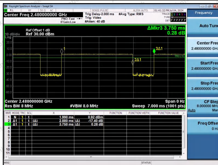
NTNV-DH5-Ant1-2480
