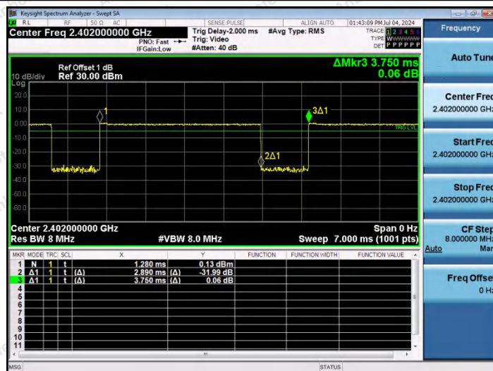
NTNV-2DH5-Ant1-2402
