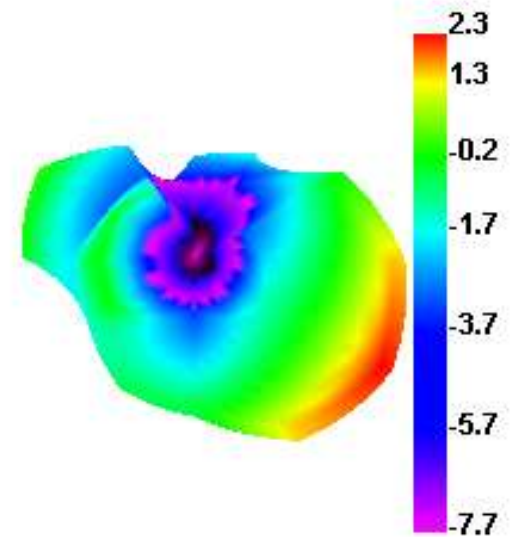
2480.000MHz
