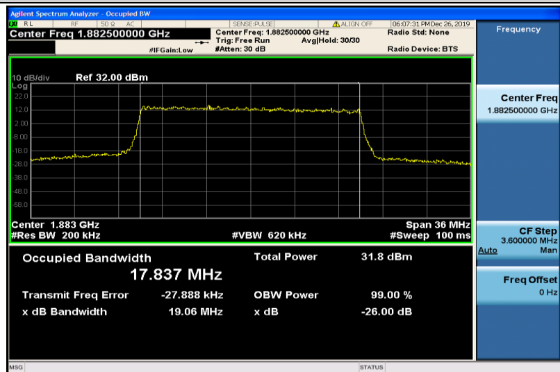
Band25-20MHz-QPSK-26365-100RB#0-17.837
