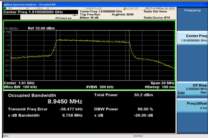
Band25-10MHz-QPSK-26640-50RB#0-8.9450
