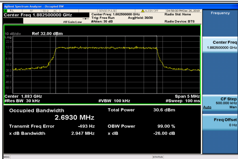
Band25-3MHz-QPSK-26365-15RB#0-2.6930
