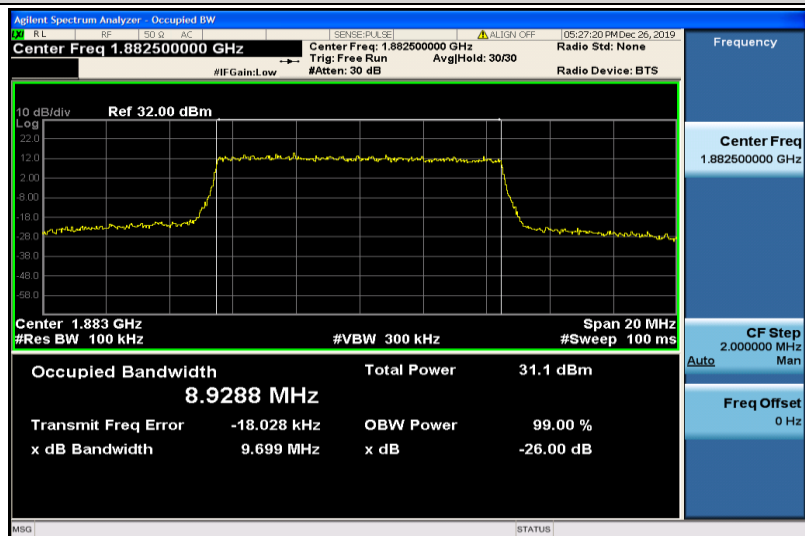
Band25-10MHz-QPSK-26365-50RB#0-8.9288
