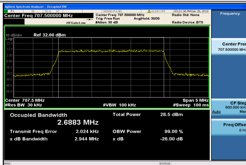
Band12-3MHz-QPSK-23095-15RB#0-2.6883
