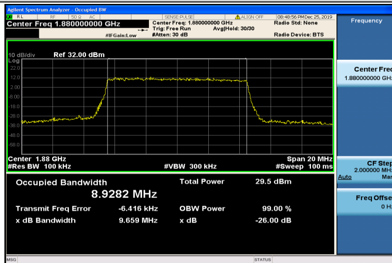
Band2-10MHz-16QAM-18900-50RB#0-8.9282
