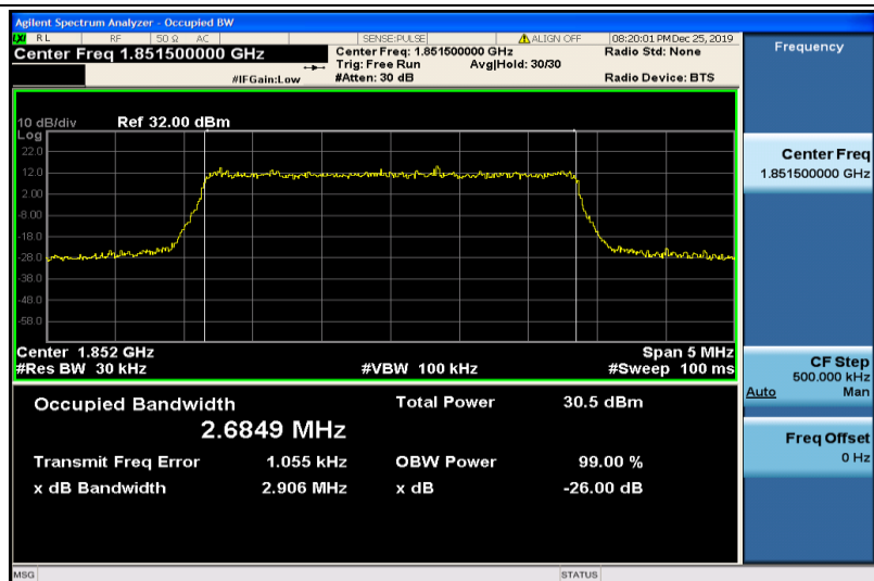
Band2-3MHz-QPSK-18615-15RB#0-2.6849
