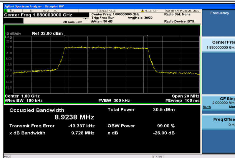
Band2-10MHz-QPSK-18900-50RB#0-8.9238
