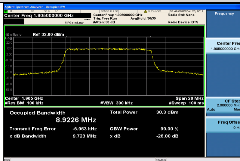
Band2-10MHz-QPSK-19150-50RB#0-8.9226
