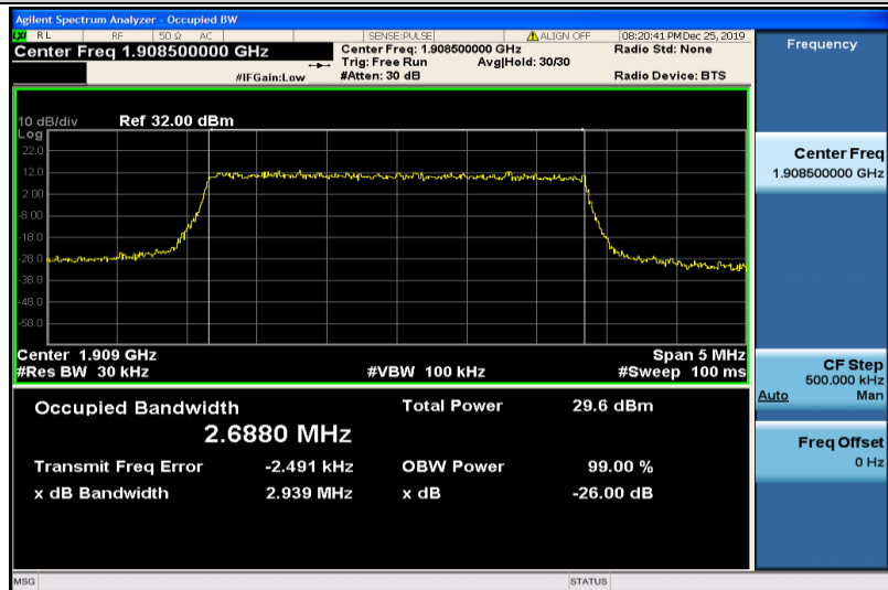
Band2-3MHz-QPSK-19185-15RB#0-2.6880
