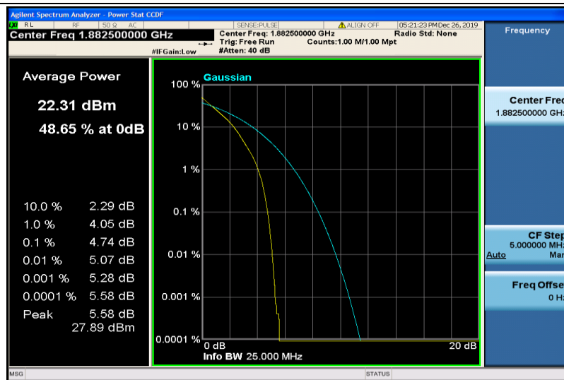
Band25-5MHz-QPSK-26365-25RB#0
