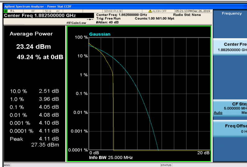
Band25-5MHz-QPSK-26365-1RB#0
