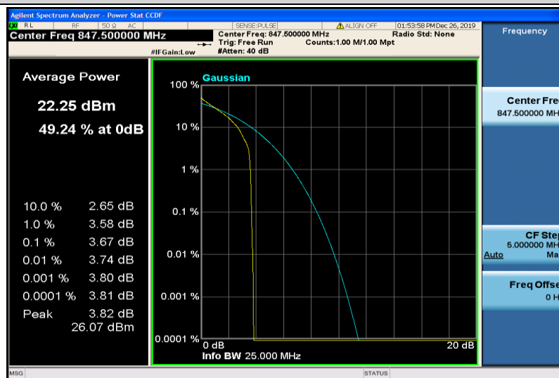
Band5-3MHz-QPSK-20635-1RB#0
