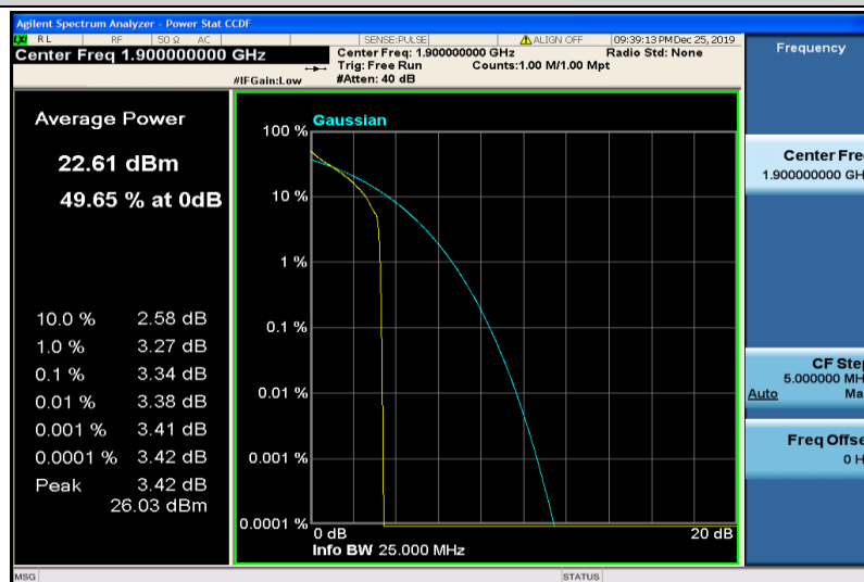
Band2-20MHz-QPSK-19100-1RB#0
