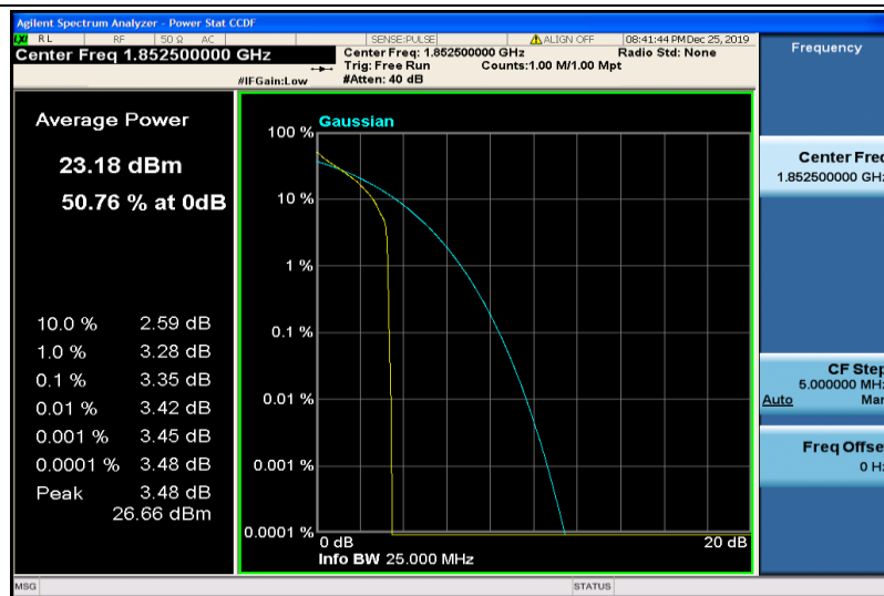
Band2-5MHz-QPSK-18625-1RB#0
