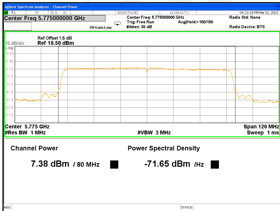
5775MHz_AV_Ant A
