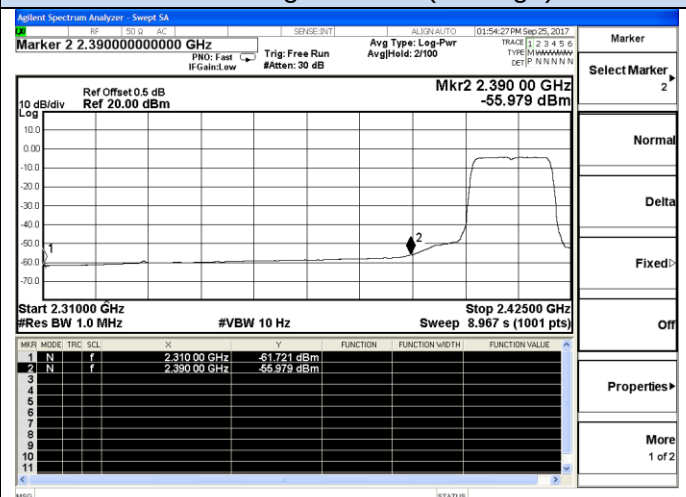
802.11g-Low channel(Average)
