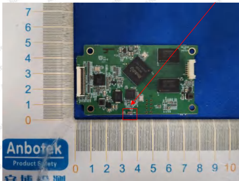
BLE 1 Antenna
