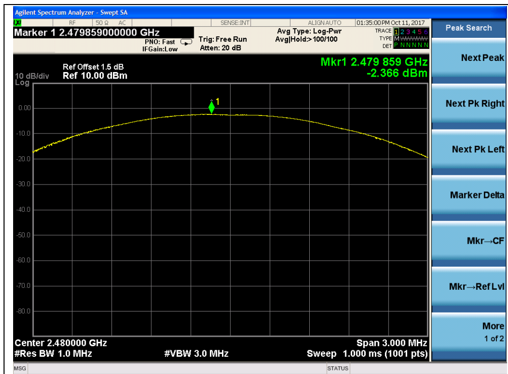
(Channel 39, 2480MHz, \pi/4 -DQPSK)
