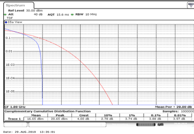
Band2_15MHz_QPSK_18900_75RB#0
