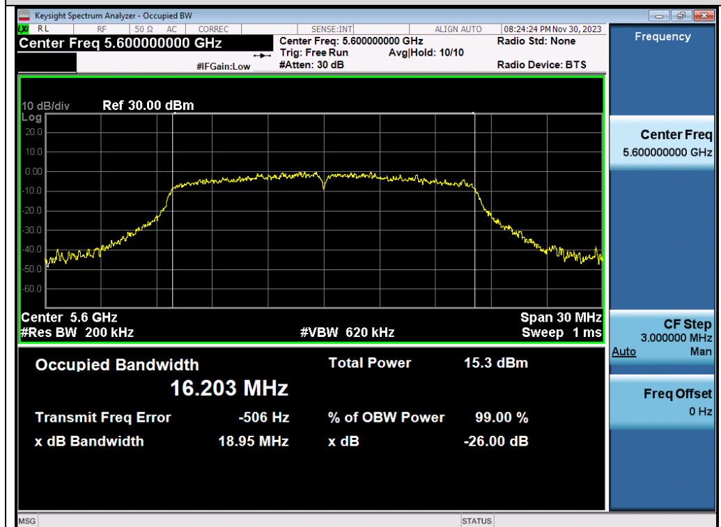
Test_Graph_802.11a_ANT1_5600_6Mbps_OBW
