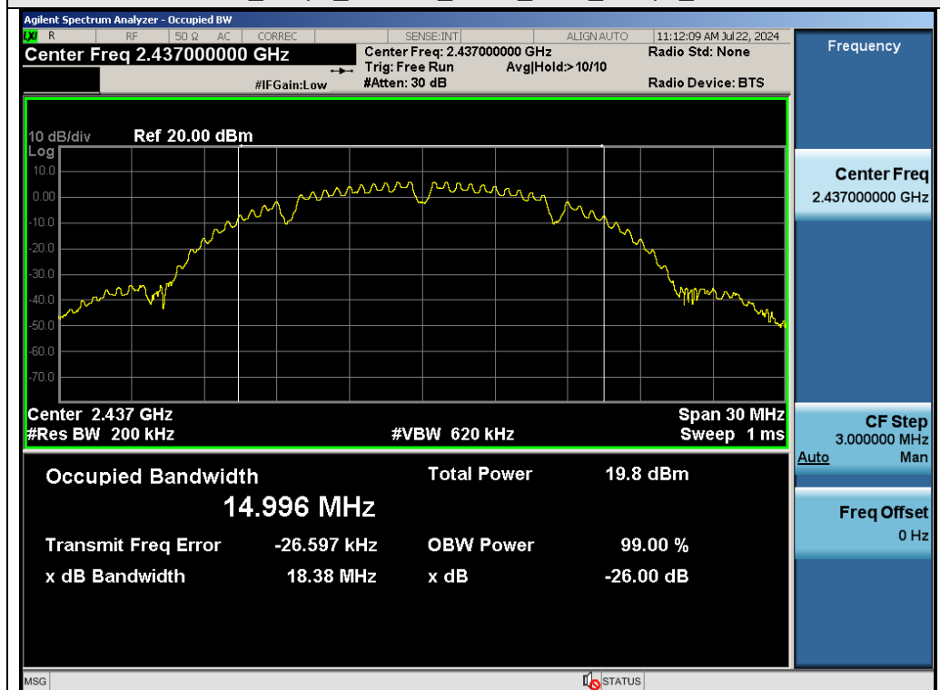
Test_Graph_802.11b_ANTA_2437_1Mbps_OBW
