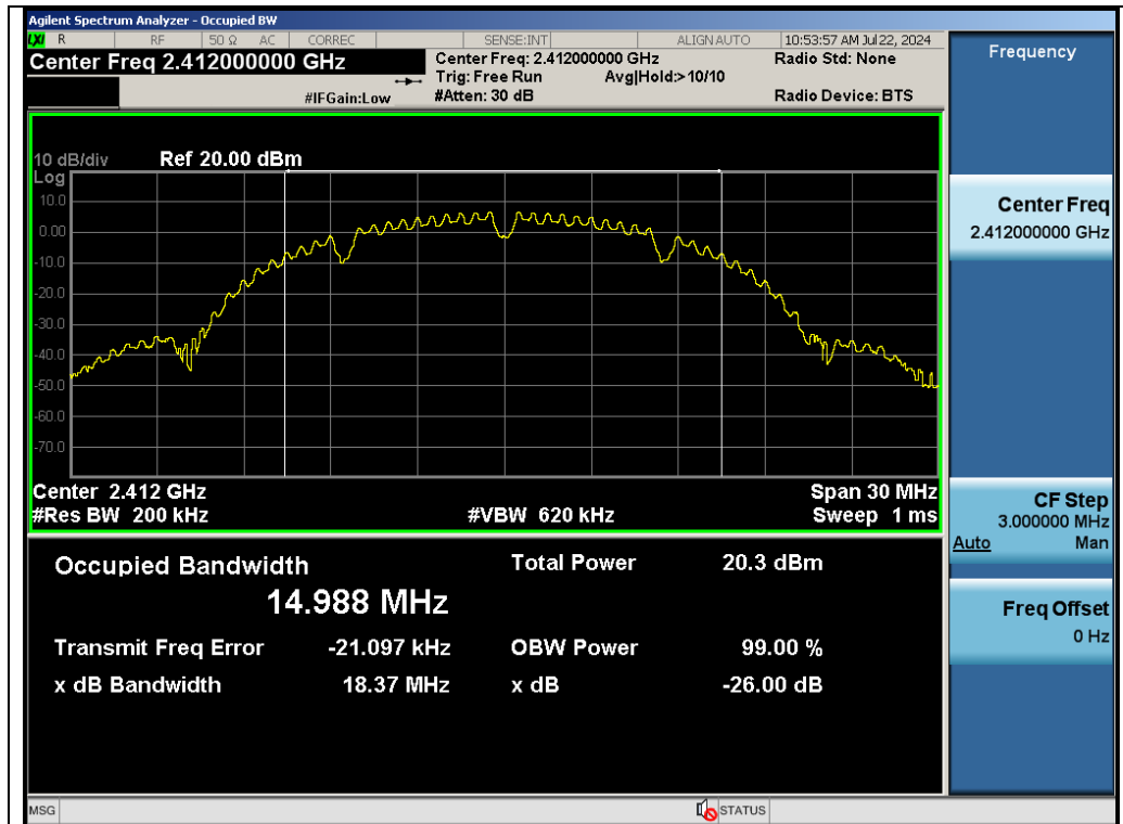
Test_Graph_802.11b_ANTA_2412_1Mbps_OBW
