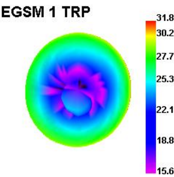
EGSM 1 TRP
