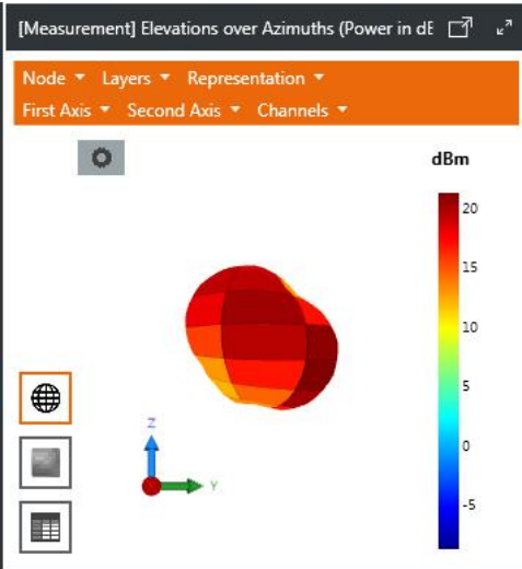
LTE B20 TRP
