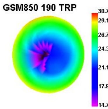
GSM850 190 TRP
