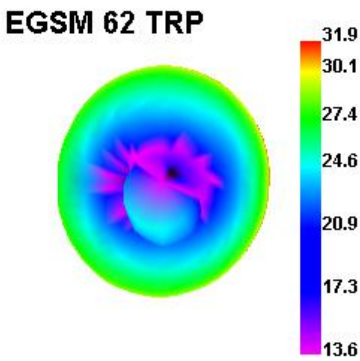
EGSM 62 TRP
