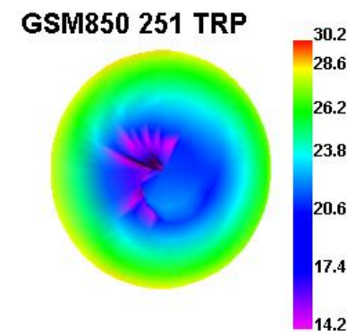
GSM850 251 TRP
