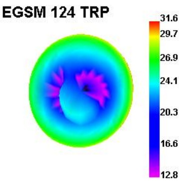
EGSM 124 TRP
