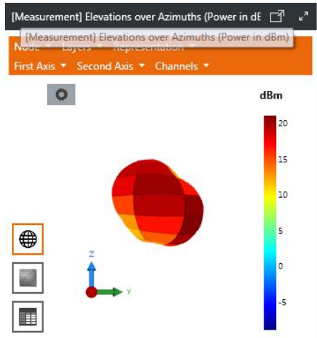
LTE B5 TRP
