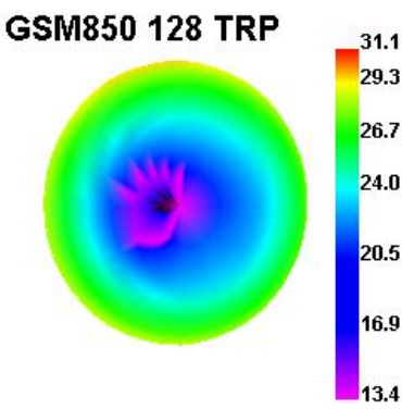
GSM850 128 TRP
