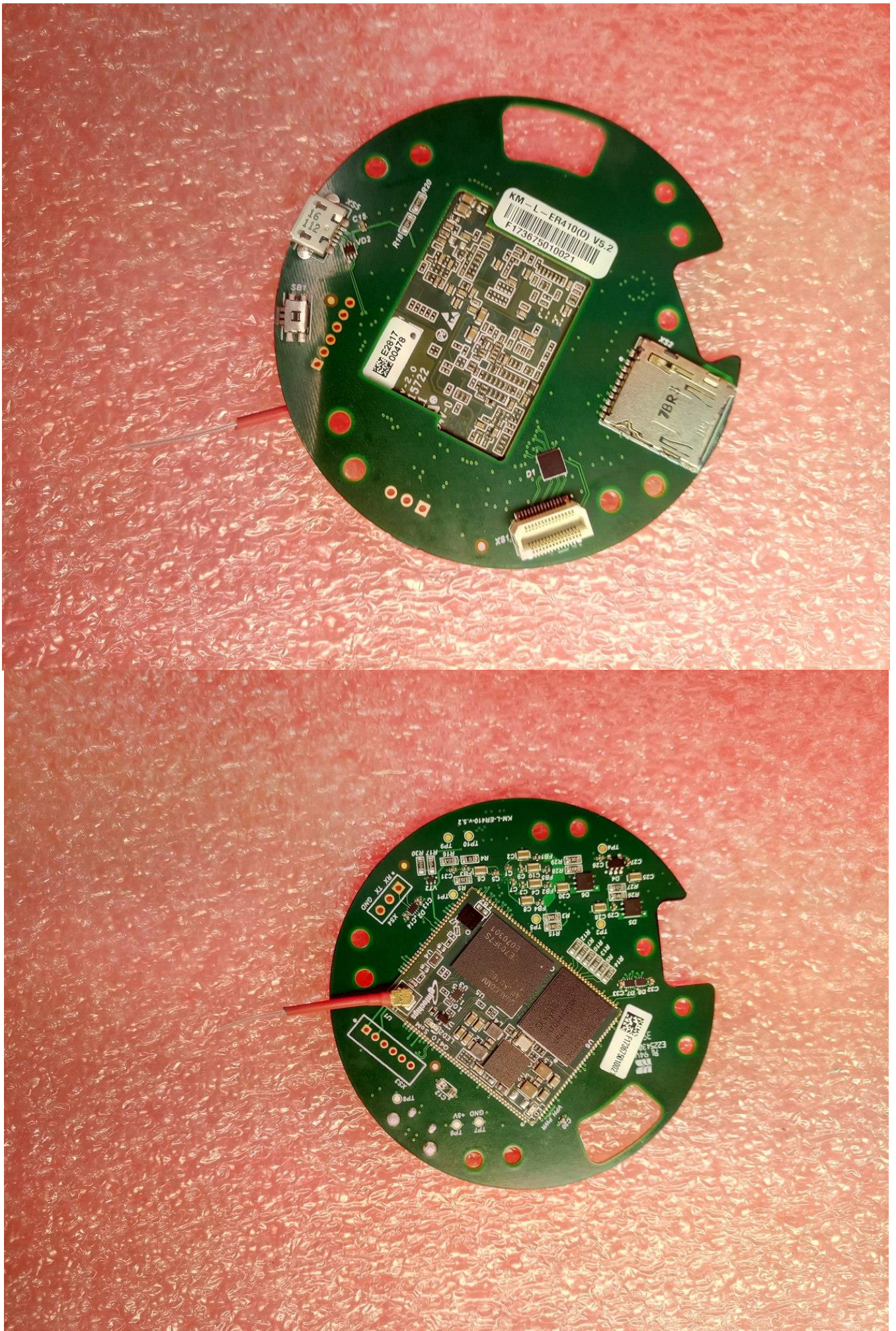
Fig. 1. KM-L-ER410
