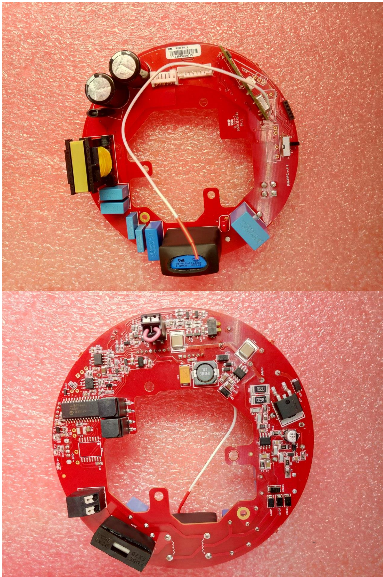
Fig 5. KM-PFC
