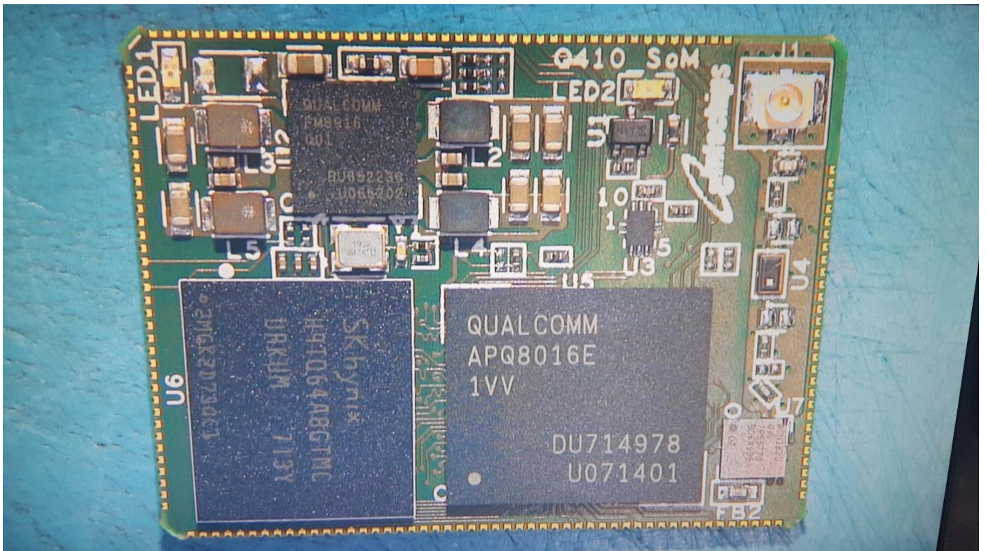
Fig. 1.1 Eragon 410 SOM
