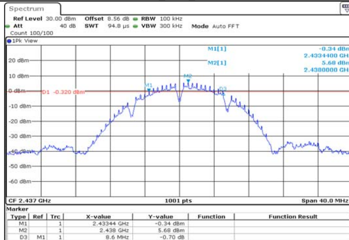
11B_Ant1_2437
