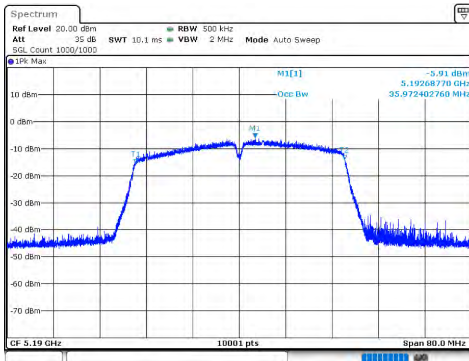
OBW NVNT 802.11ac40 5190MHz Ant1
