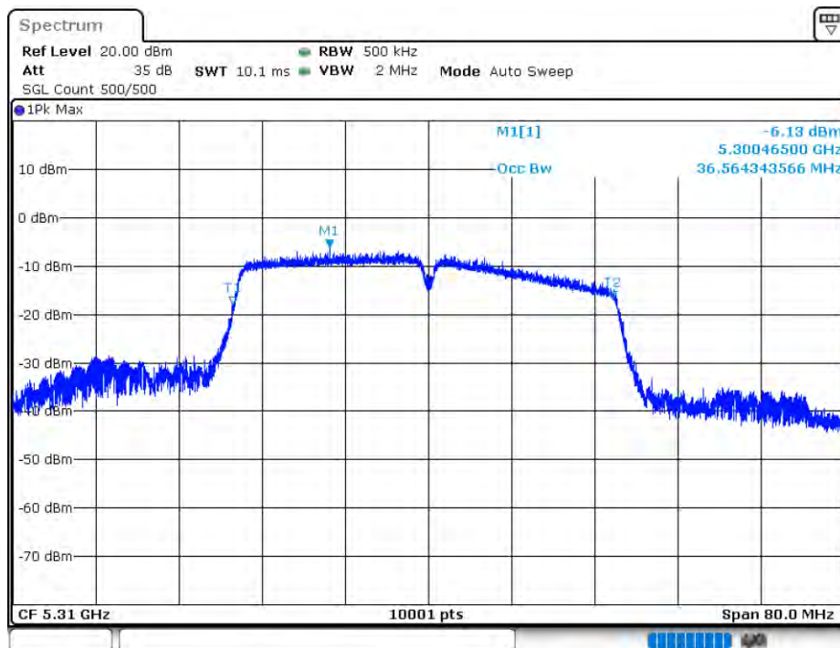
OBW NVNT 802.11n(HT40) 5310MHz Ant1
