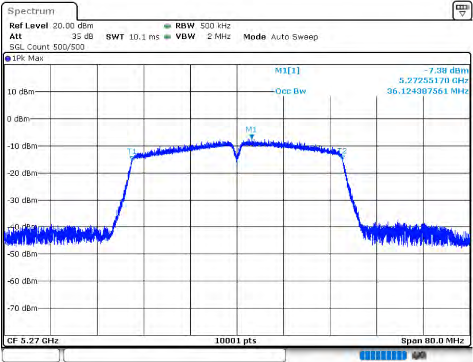
OBW NVNT 802.11n(HT40) 5270MHz Ant1
