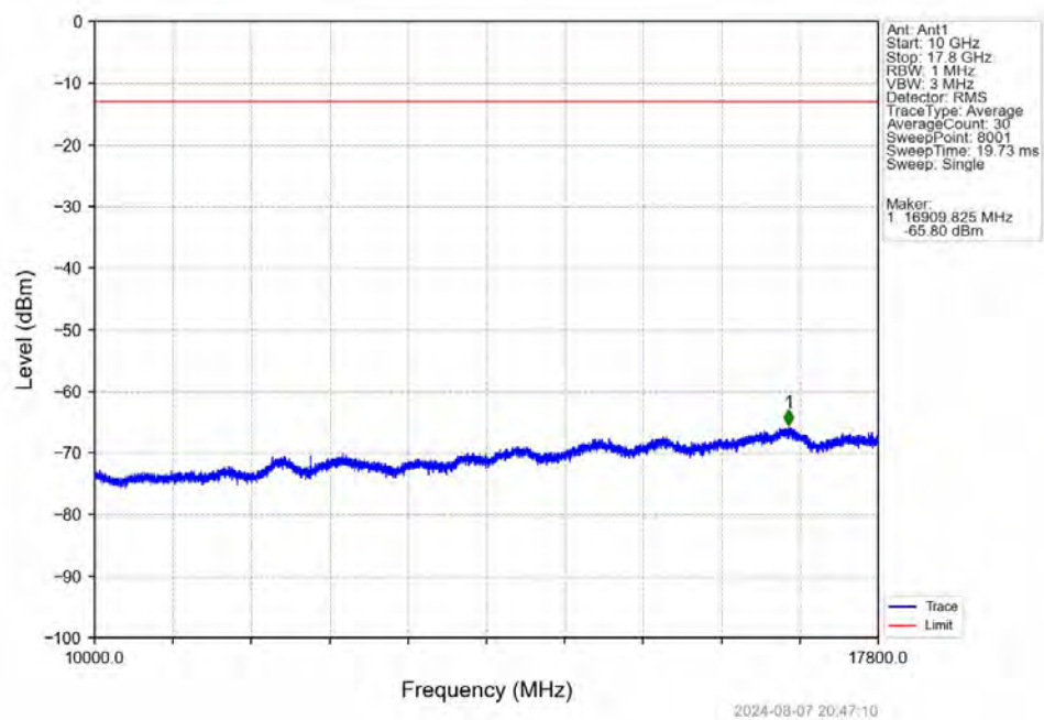
Band66_20MHz_QPSK_MCH_1745MHz_RB_1_0_NTNV
