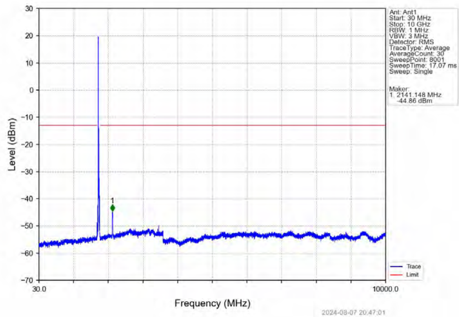
Band66_20MHz_QPSK_MCH_1745MHz_RB_1_0_NTNV
