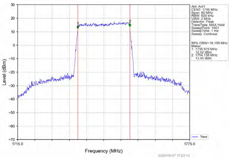
Band66_20MHz_QPSK_MCH_1745MHz_RB_100_0_NTNV
