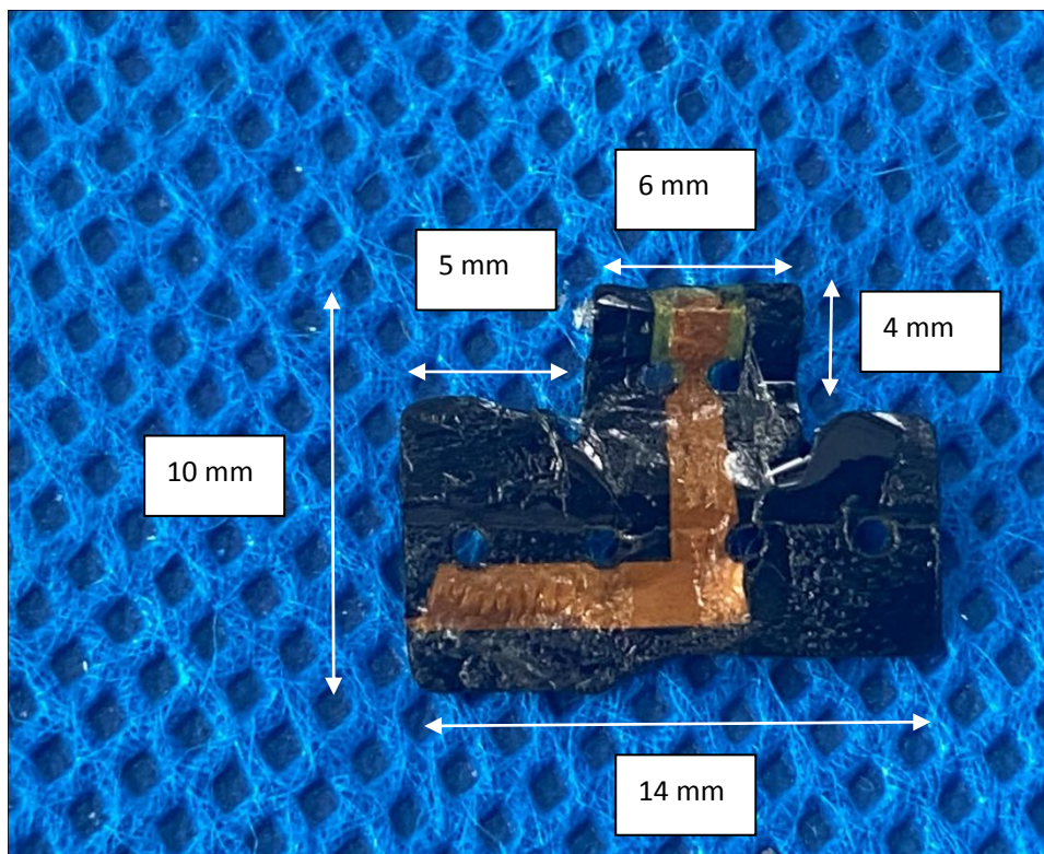
BT&WIFI 2.4G/5G antenna
