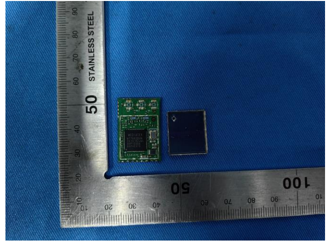
EUT
