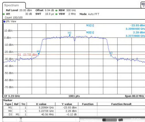
11AC40MIMO-Ant1-5230
