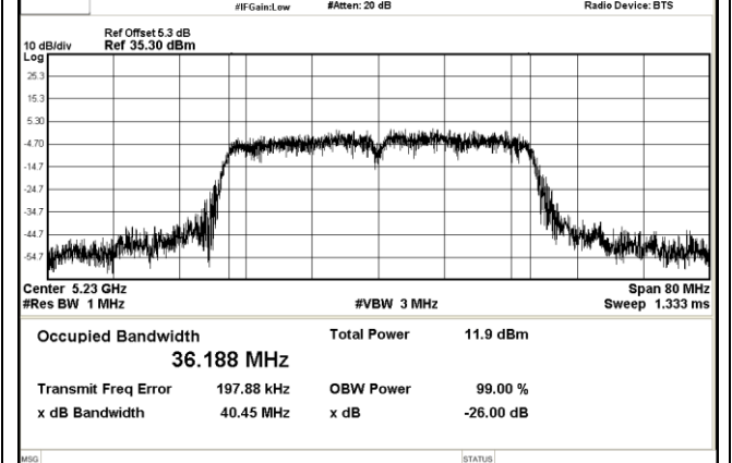
ANT 2
