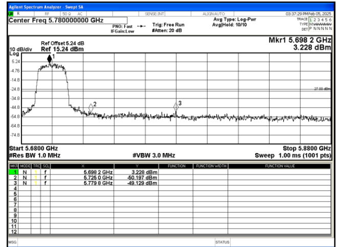
802.11 n20 5700MHz
