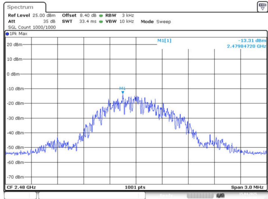
PSD NVNT BLE 1M 2480MHz Ant1
