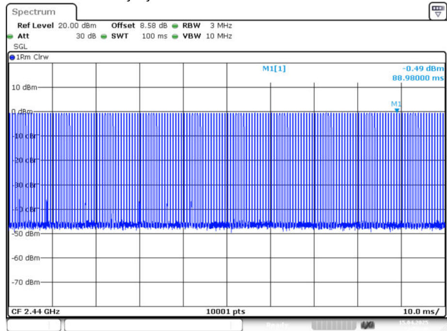
Duty Cycle NVNT BLE 1M 2440MHz Ant1
