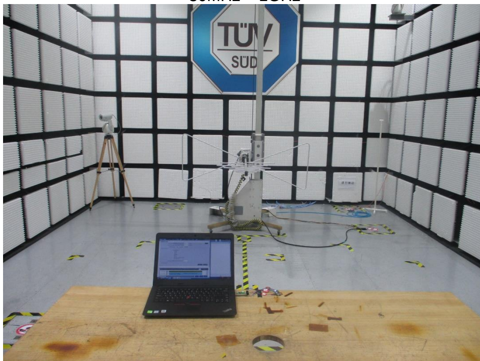
30MHz ~ 1GHz
