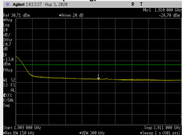
RB(Starting):0 RB#100
