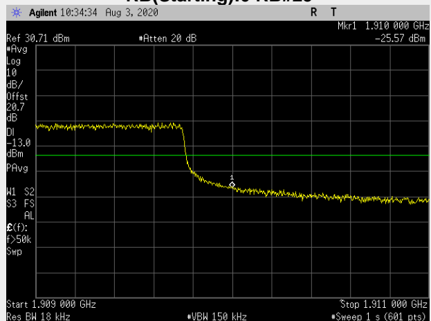
RB(Starting):0 RB#25
