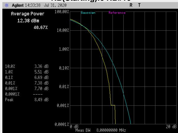
RB(Starting):0 RB#16
