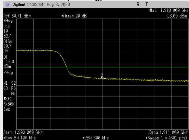
RB(Starting):0 RB#50
