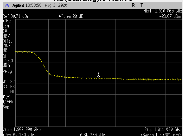
RB(Starting):0 RB#75
