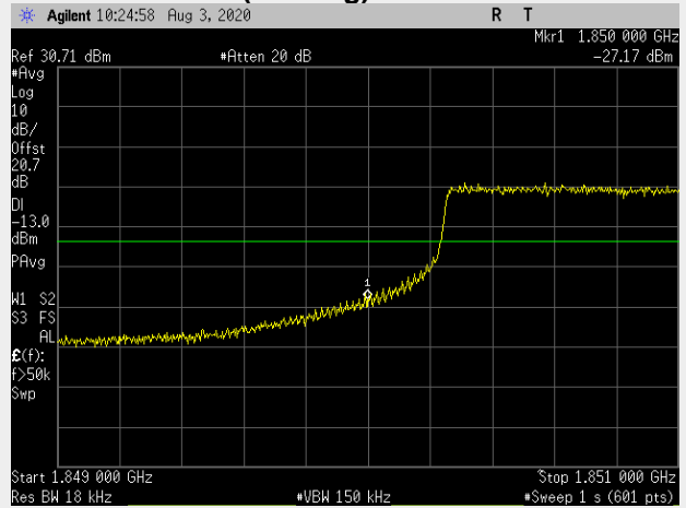
RB(Starting):0 RB#25
