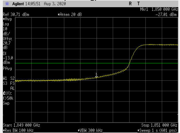
RB(Starting):0 RB#50
