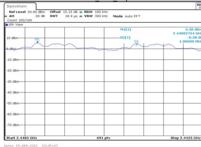
3DH1_Ant1_Hop
