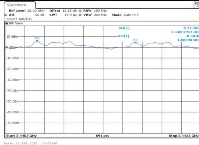
3DH1_Ant1_Hop
