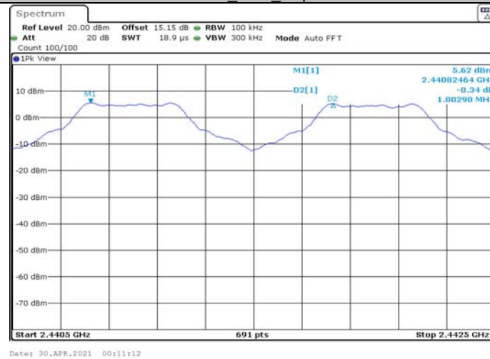
2DH1_Ant1_Hop
