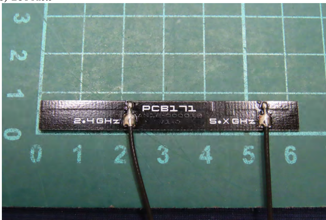
(9) EUT Photo
