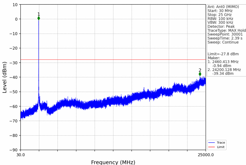
802.11n(HT20)_HCH_2462MHz_Ant0 (MIMO)_NTNV
