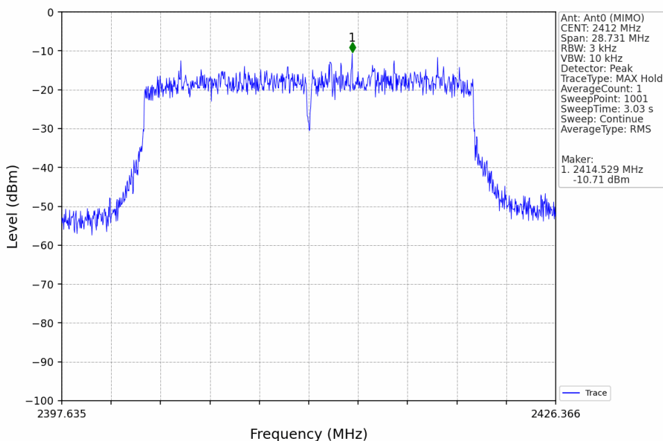
802.11ax(HEW20)_LCH_2412MHz_RU242_Left_Ant0 (MIMO)_NTNV
