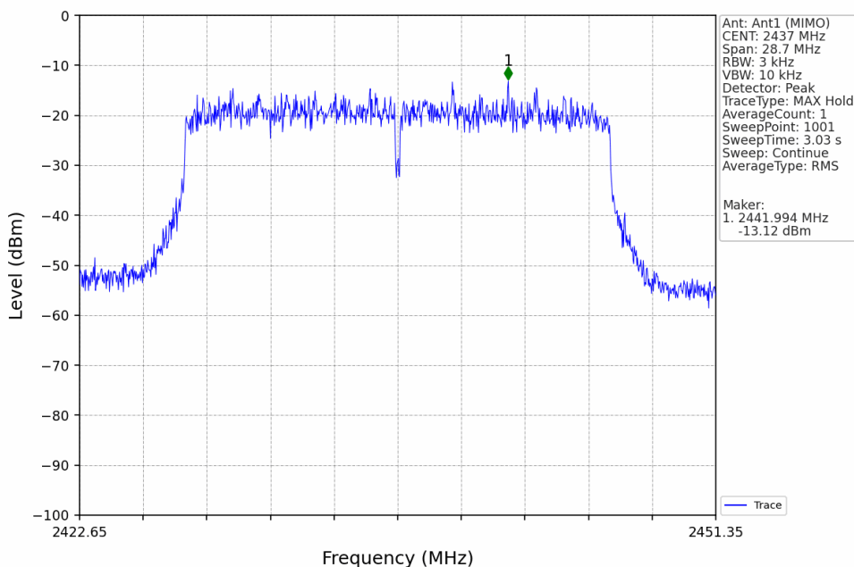
802.11ax(HEW20)_MCH_2437MHz_RU242_Left_Ant1 (MIMO)_NTNV
