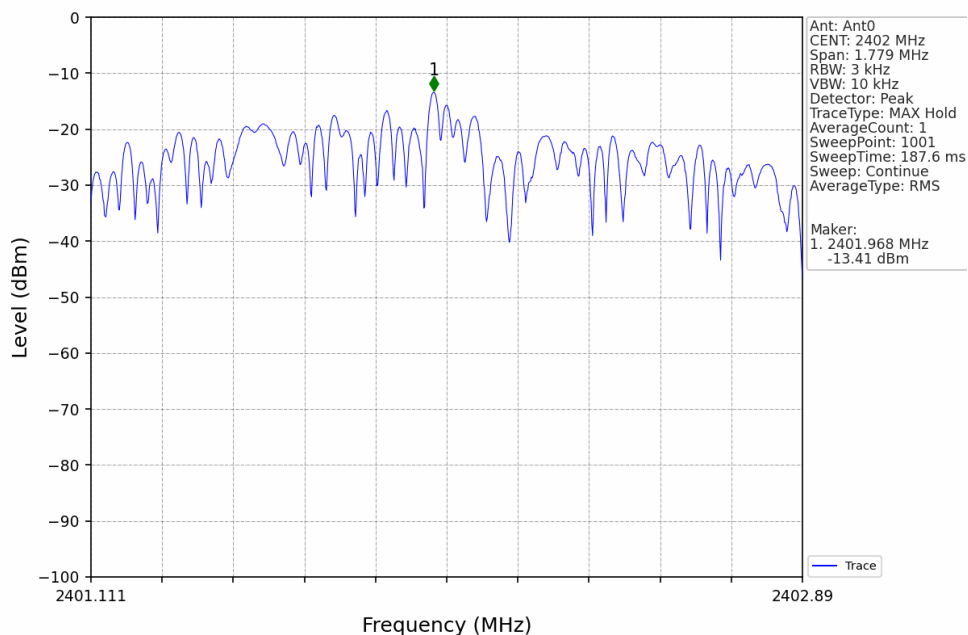
2M_LCH_2402MHz_Ant0_NTNV
