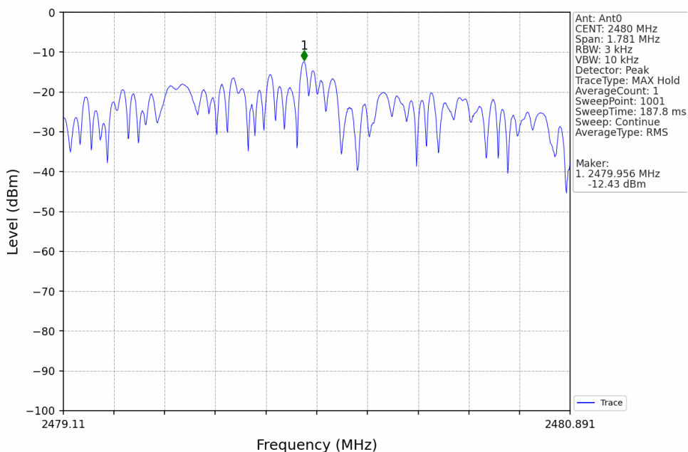
2M_HCH_2480MHz_Ant0_NTNV
