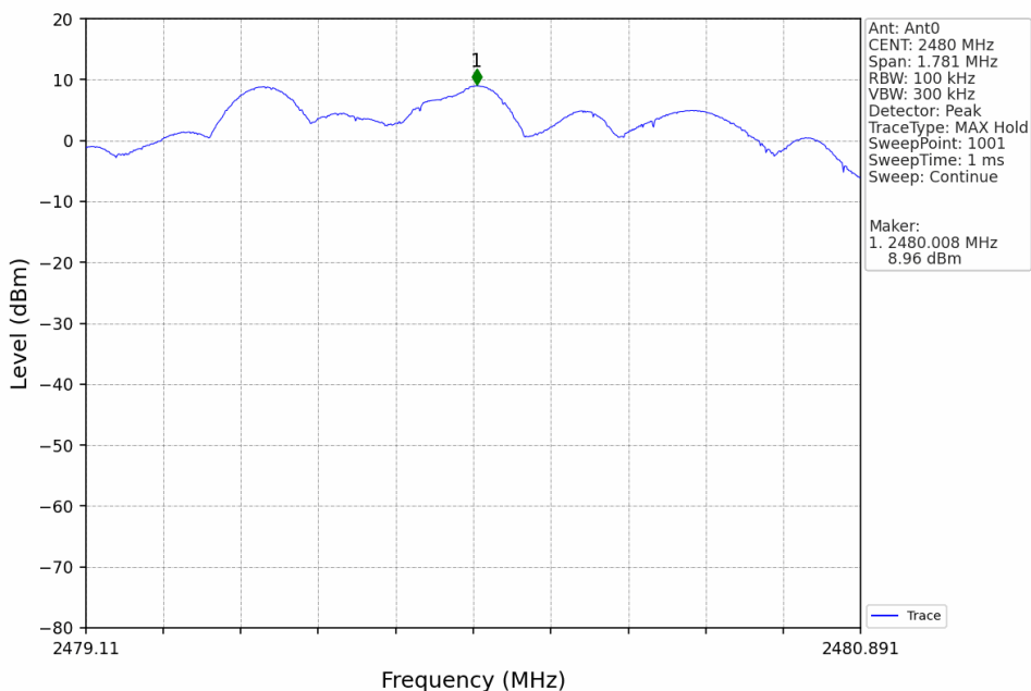
2M_HCH_2480MHz_Ant0_NTNV
