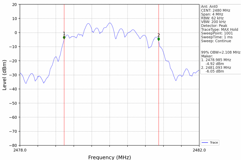
2M_HCH_2480MHz_Ant0_NTNV
