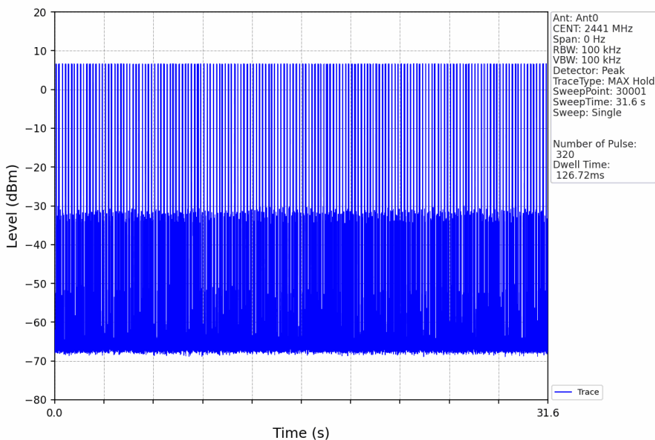
Pi/4DQPSK_2DH1_HOPP_Ant0_NTNV
