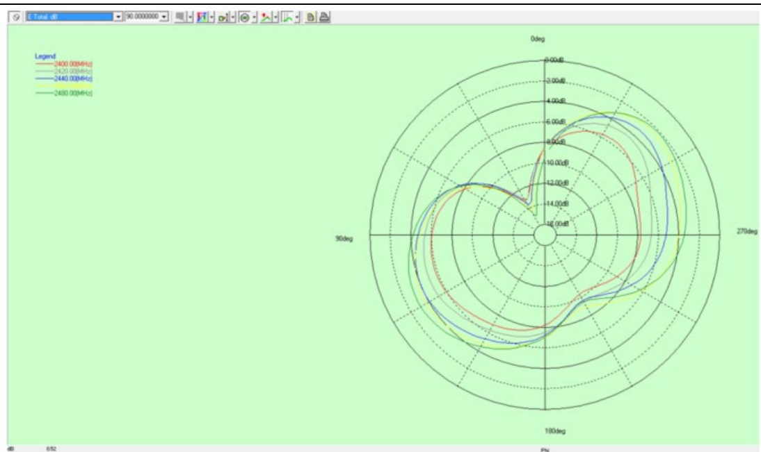
2.4G 俯仰面
