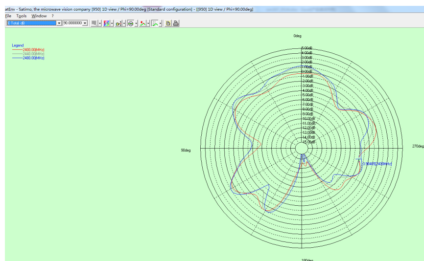
俯仰面 \phi=90^\circ
