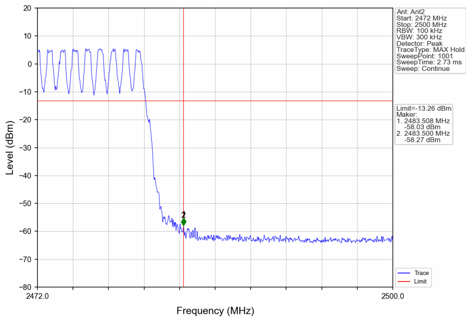
GFSK_DH5_HOPP_Ant2_NTNV
