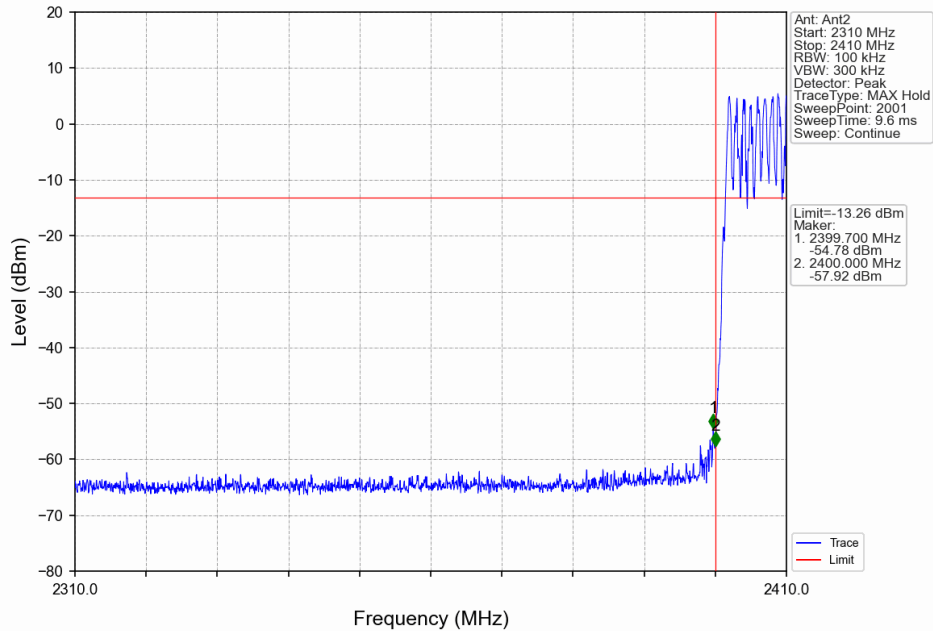
GFSK_DH5_HOPP_Ant2_NTNV
