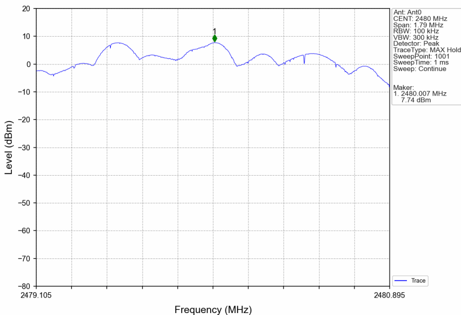
2M_HCH_2480MHz_Ant0_NTNV
