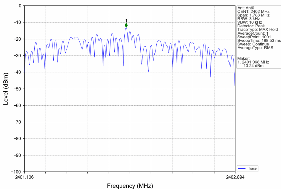
2M_LCH_2402MHz_Ant0_NTNV
