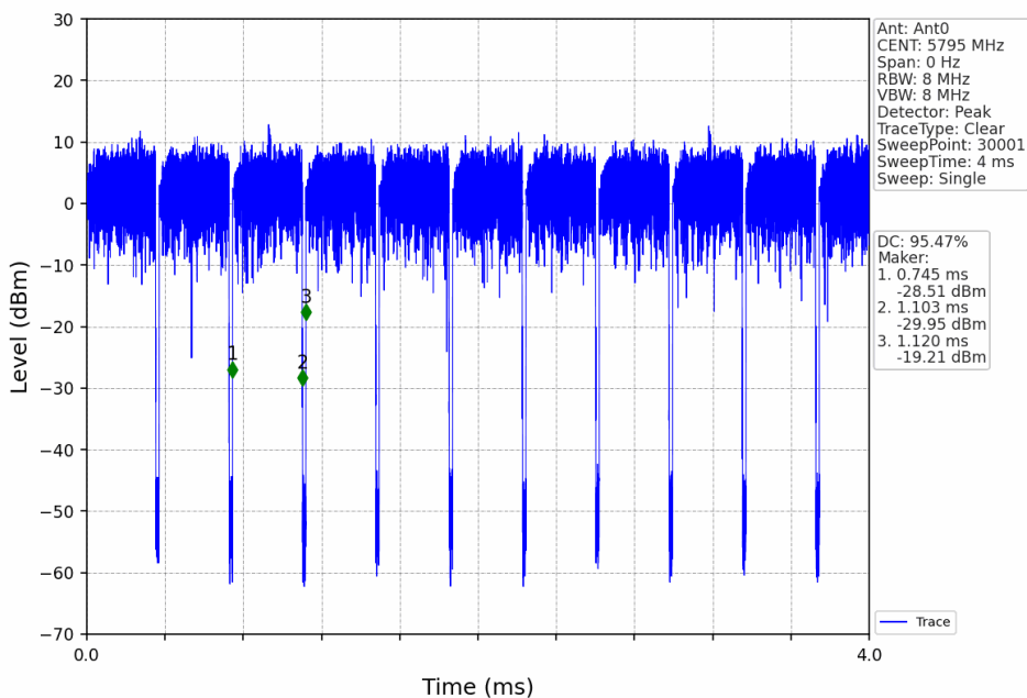
802.11n(HT40)_HCH_5795MHz_Ant0_NTNV
