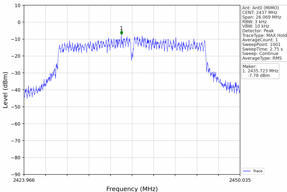
802.11n(HT20)_MCH_2437MHz_Ant0 (MIMO)_NTNV
