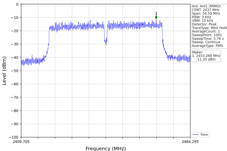
802.11n(HT40)_MCH_2437MHz_Ant1 (MIMO)_NTNV
