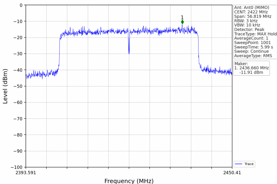
802.11ax(HEW40)_LCH_2422MHz_RU484_Left_Ant0 (MIMO)_NTNV
