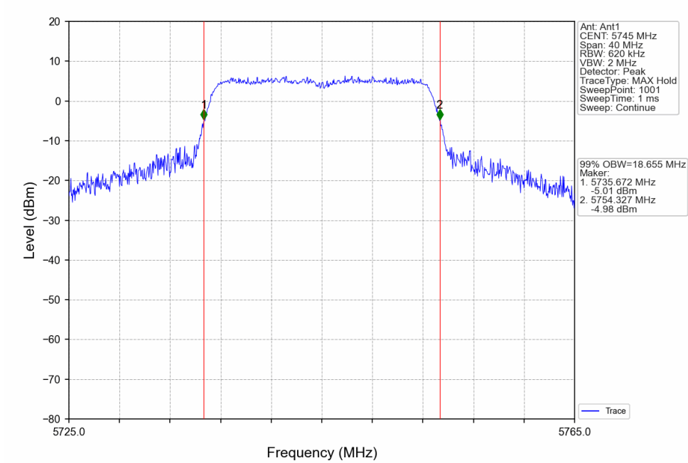
802.11n(HT20)_LCH_5745MHz_Ant1_NTNV
