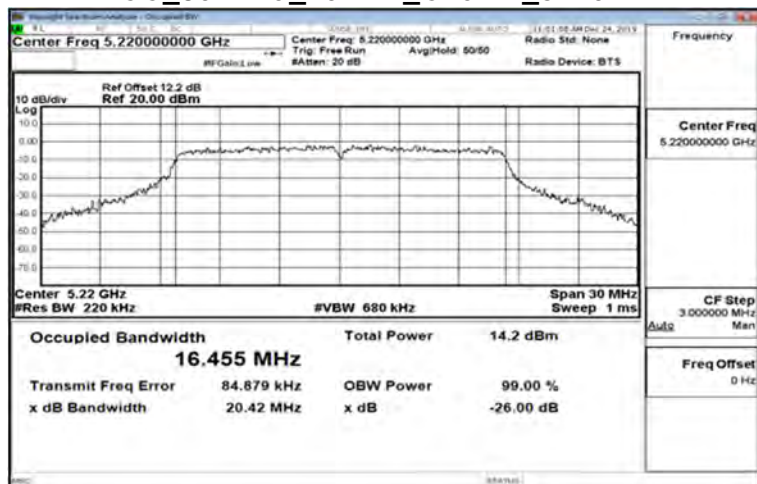
FCC_802.11a_20MHz_Chain1_5220MHz
