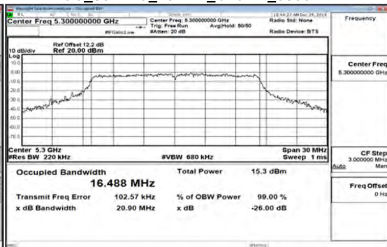
FCC_802.11a_20MHz_Chain1_5300MHz
