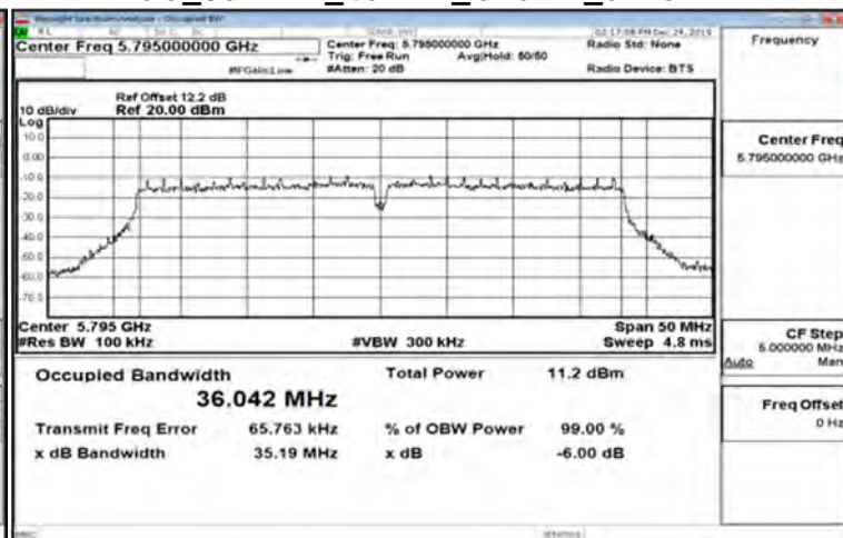
FCC_802.11n_40MHz_Chain1_5795MHz
