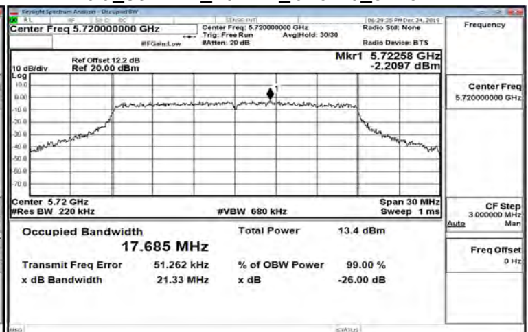
FCC_802.11n_20MHz_Chain0_5720MHz
