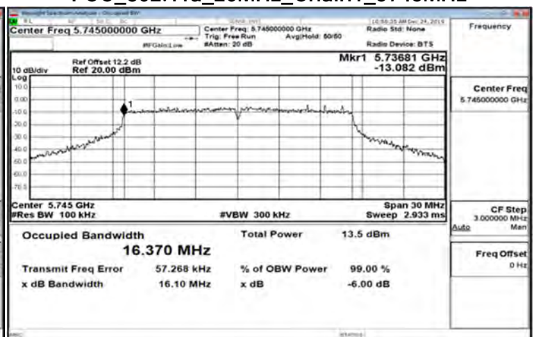
FCC_802.11a_20MHz_Chain1_5745MHz
