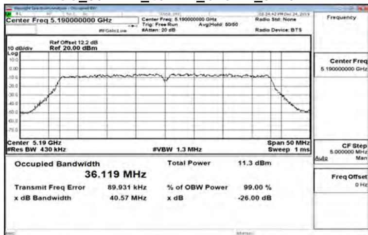
FCC_802.11n_40MHz_Chain1_5190MHz
