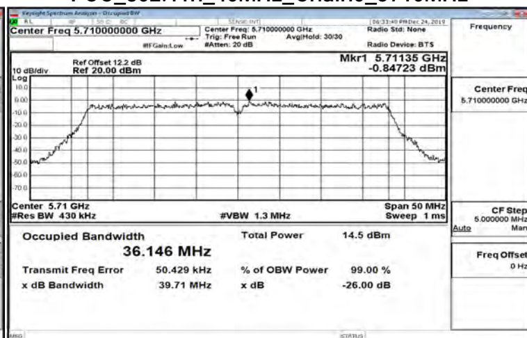
FCC_802.11n_40MHz_Chain0_5710MHz
