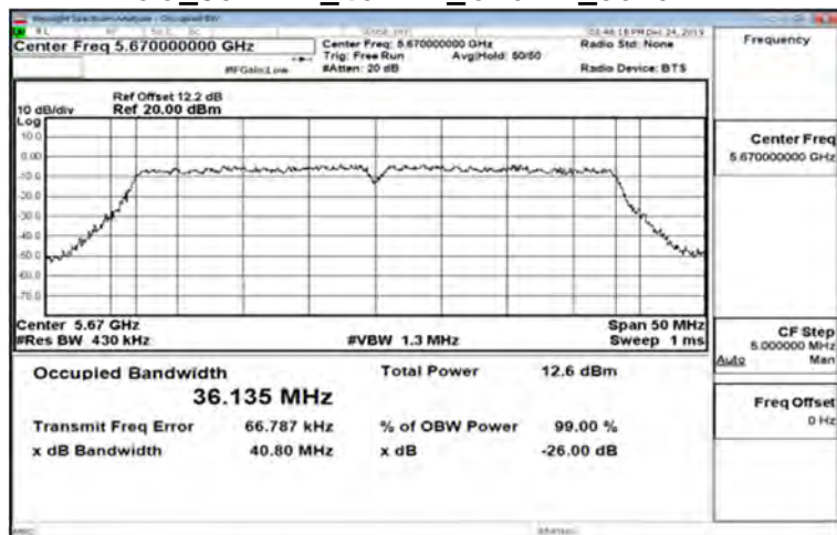
FCC_802.11n_40MHz_Chain1_5670MHz
