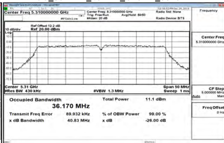
FCC_802.11n_40MHz_Chain1_5310MHz
