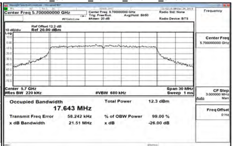
FCC_802.11n_20MHz_Chain1_5700MHz
