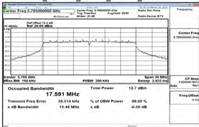
FCC_802.11n_20MHz_Chain1_5785MHz
