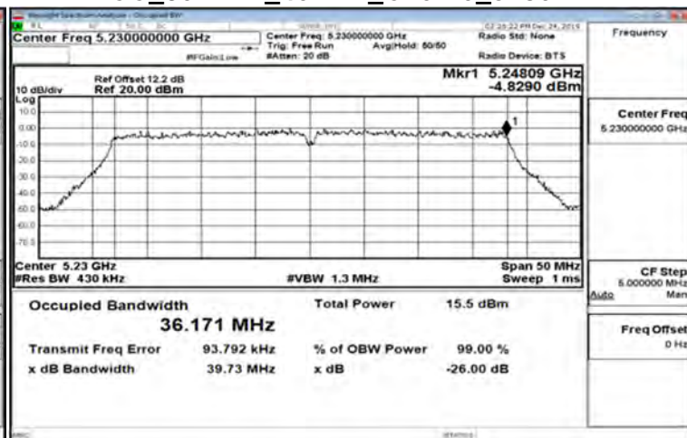
FCC_802.11n_40MHz_Chain0_5230MHz
