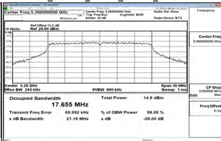
FCC_802.11n_20MHz_Chain0_5260MHz
