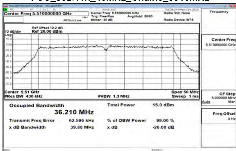
FCC_802.11n_40MHz_Chain0_5510MHz
